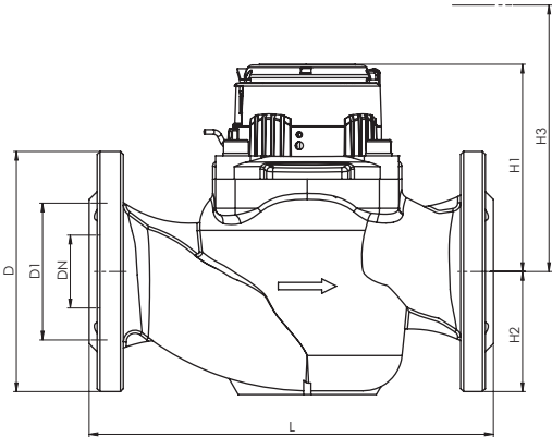
Abmessungen
