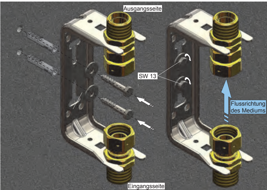
Montageschritt 3
