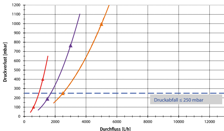
Druckverlustdiagramm
